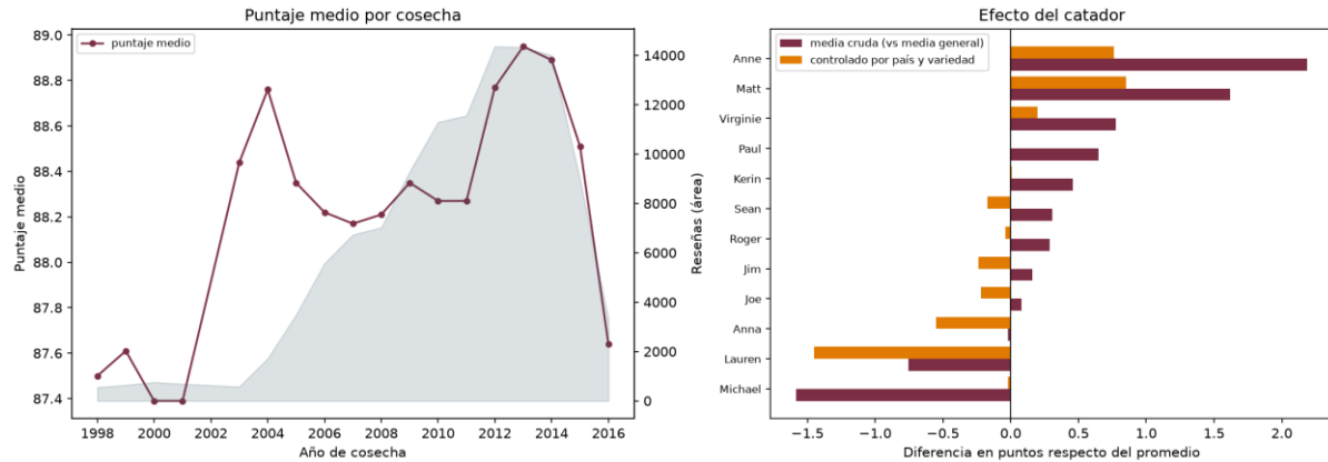
Figura 8. Puntaje medio por cosecha y cantidad de reseñas (izquierda). Efecto de cada catador antes y después de controlar por país y variedad (derecha).
