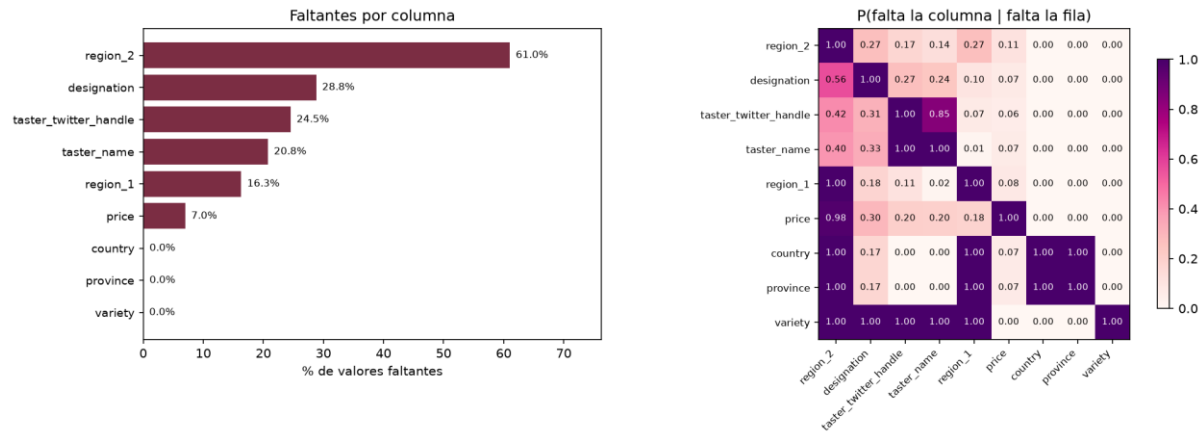
Figura 4. Porcentaje de faltantes por columna (izquierda) y probabilidad de que falte una columna dado que falta otra (derecha).
